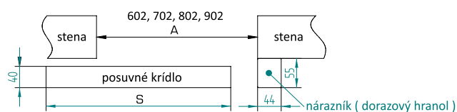
posuvný systém bez obložky „bezobložkový „
