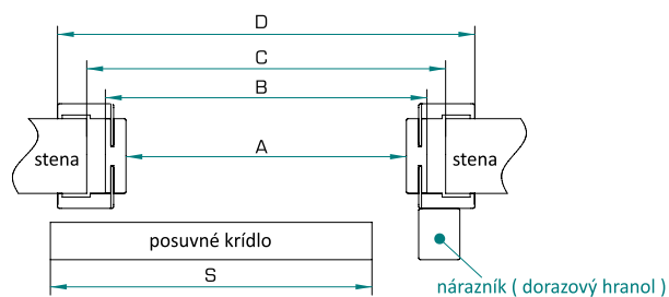
Posuvný systém s obložkovou zárubňou „tunel „
