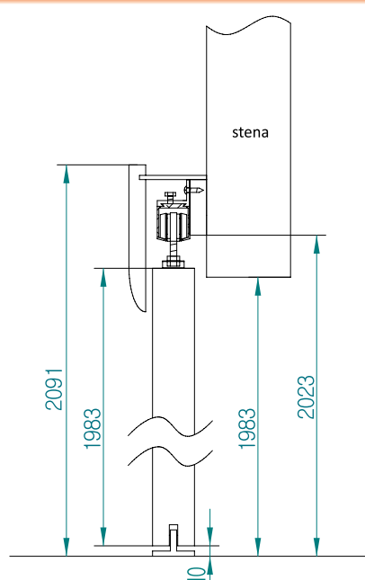
posuvný systém bez obložky „bezobložkový „
