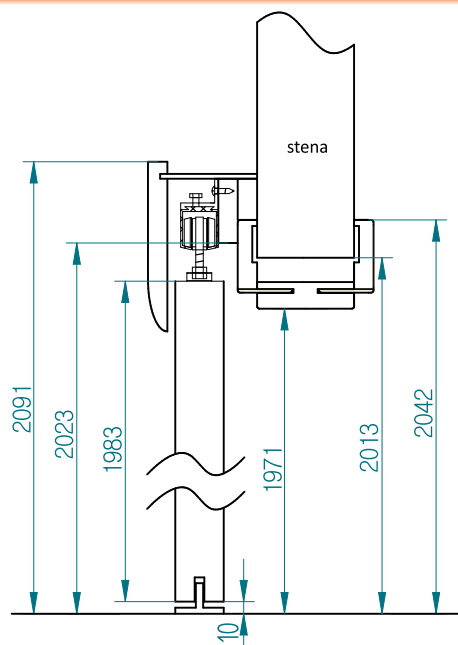
Posuvný systém s obložkovou zárubňou „tunel „
