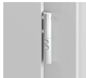
Čepové panty Ø16, nastavitelné 3D, šroubovací, v barvě zinek bílý, standardně montované do dveří SOLID PLUS a SILENZIO 32/31/29.
