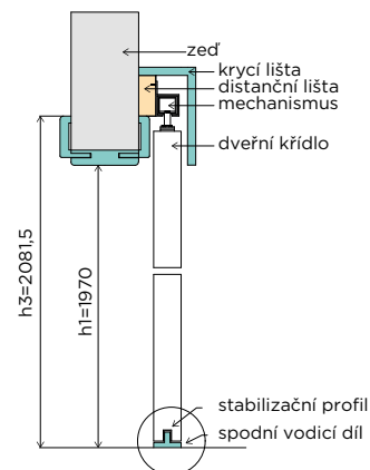
LIŠTA 100 mm H1=1970 mm
