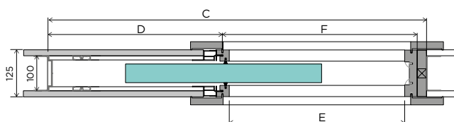
TABULKA ROZMĚRŮ PRO TLOUŠŤKU STĚNY 125 mm.
