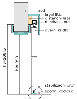
LIŠTA 60 mm H1 = 1990 mm
