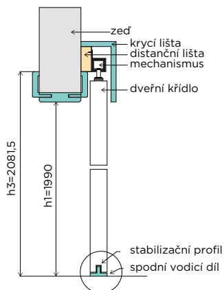
LIŠTA 80 mm H1=1990 mm
